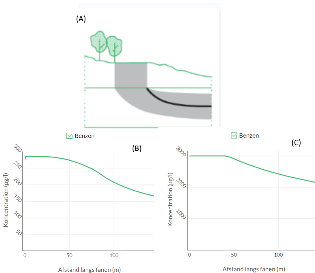
Figur 8.2 Eksempler på grafer, der viser (A) koncentrationen som funktion af afstanden fra kildeområdet. (B): Normalt kurveforløb; (C): Specialtilfælde (se afsnit 7.2.2), hvor de beregnede koncentrationer i grundvandet tæt på kilden er større end kildekonzentrationen. Her er koncentrationerne reduceret til at være lig med kildekonzentrationen. Bemærk at x = 0 svarer til den nedstrøms kant af kildeområdet.
