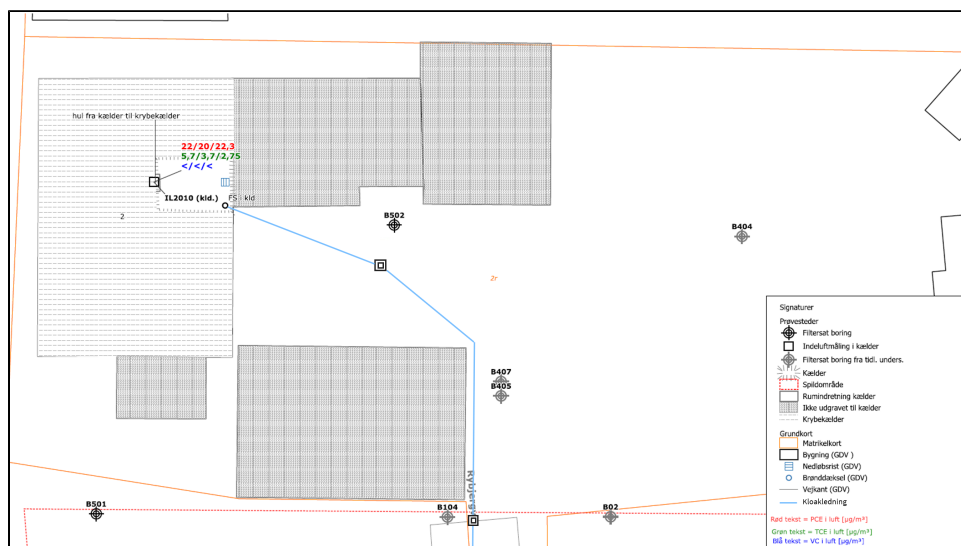
Figur 2: – viser plankort for kælder i bygningen. På kortene er påført målte koncentrationer i indeluften, samt installationer.
